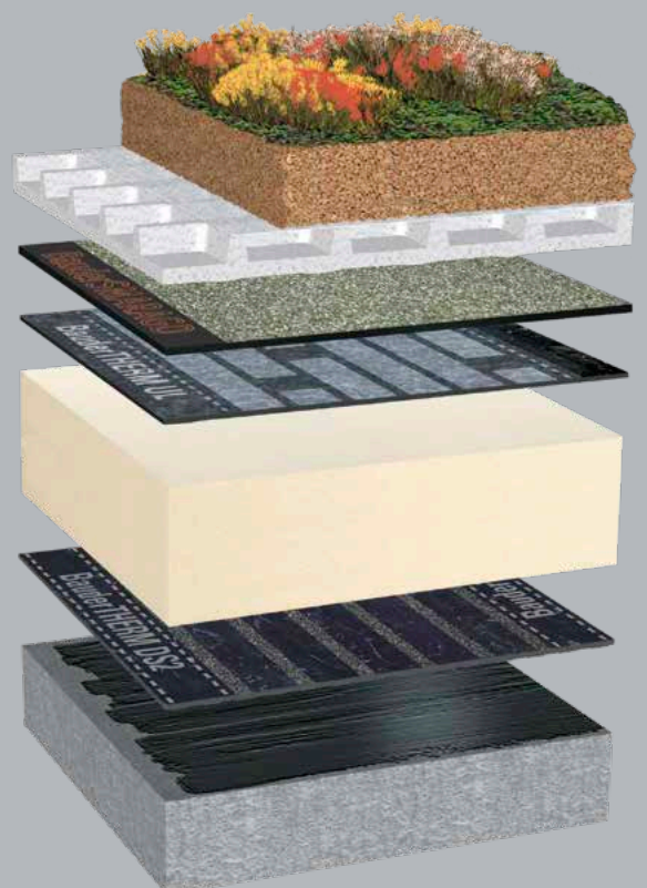
Przykład systemowego układu warstw: BauderPIR M z dwuwarstwową hydroizolacją bitumiczną oraz układem zazielenienia dachu
