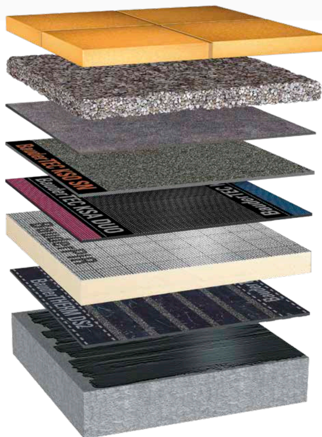
Przykład systemowego układu warstw: BauderPIR FA TE
